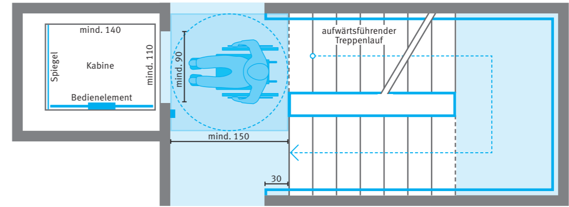
Grundrissbeispiel Aufzug und zweiläufige Treppe
