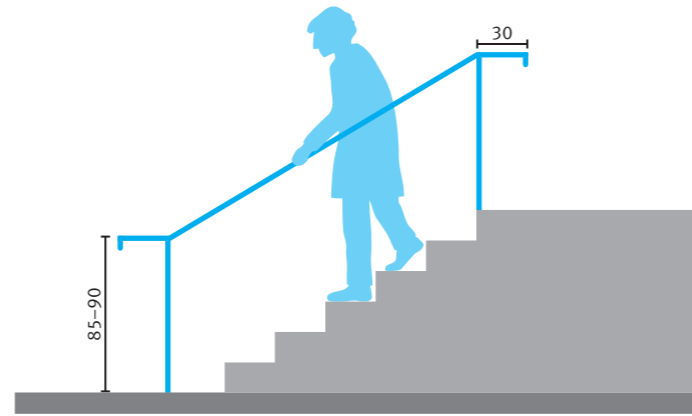
Treppe von der Seite
