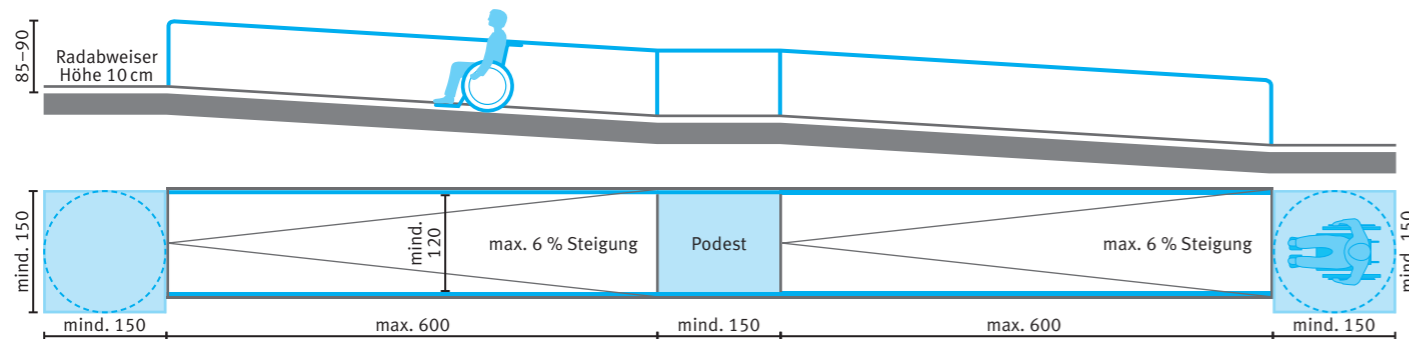
Rampe von der Seite und von oben
