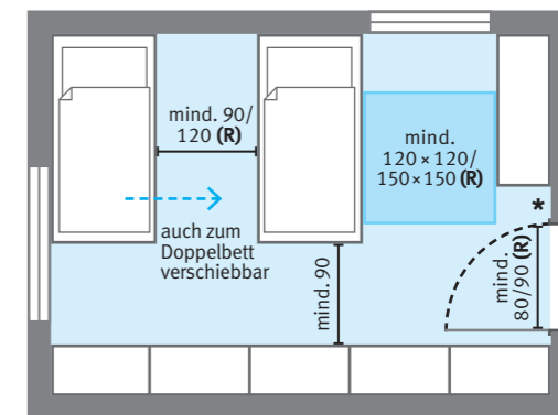
Grundrissbeispiel Schlafzimmer (Zeichnung ohne Maßstab)
