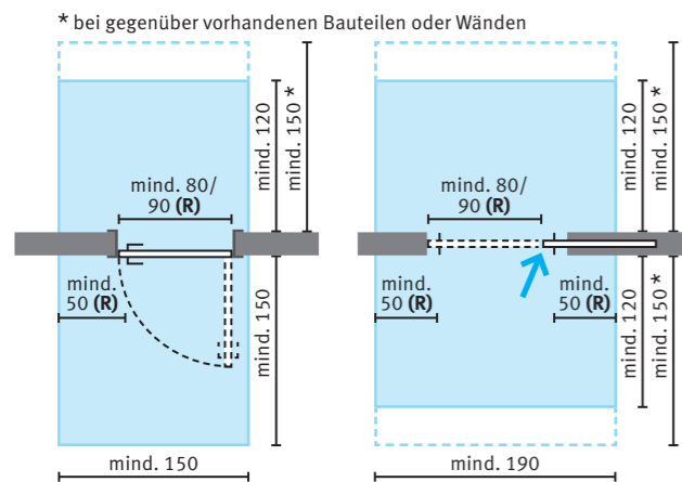
Drehflügeltür und Schiebetür (ohne Maßstab)
