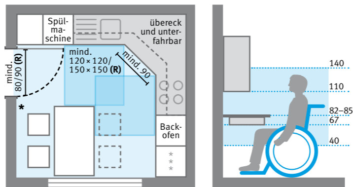
* Achtung: mindestens 50 cm Abstand bei Rollstuhl- oder Rollatornutzung Grundrissbeispiel Küche und Unterfahrbare (Zeichnungen ohne Maßstab)
