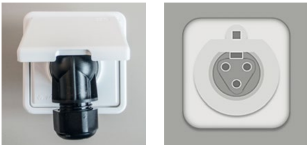
Einspeisesteckdose mit dem Spezialstecker Typ „Wieland“.
