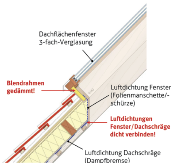
Anschlussdetail Dachflächenfenster
